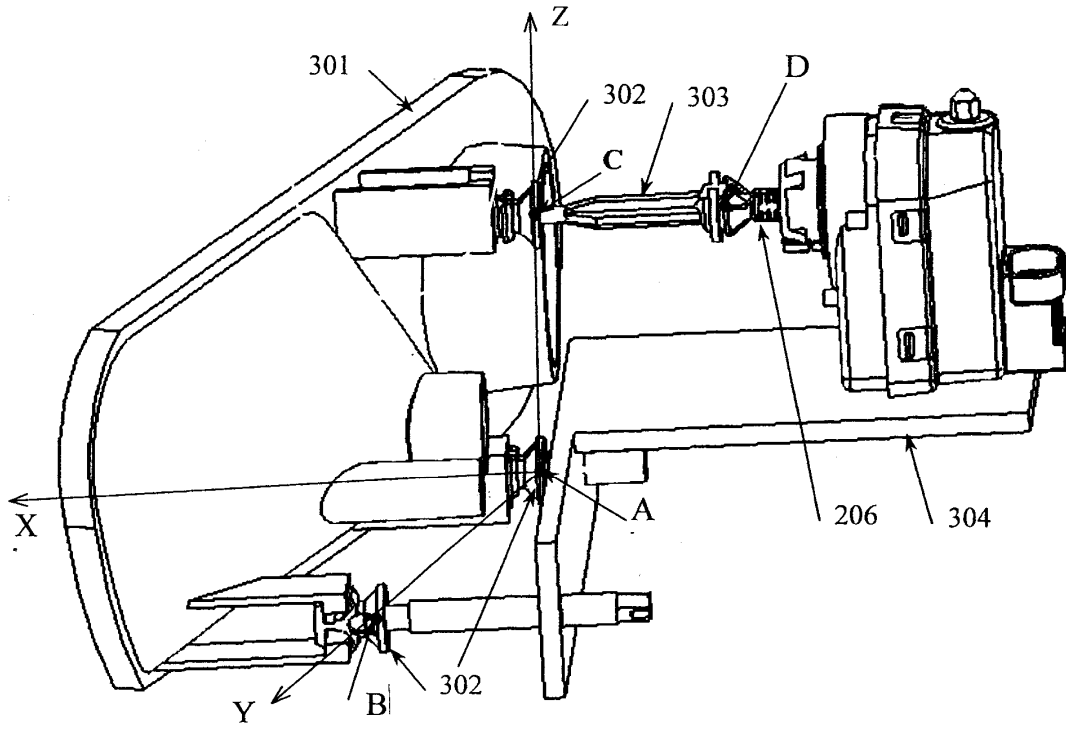
SCHÉMA CINÉMATIQUE DU BLOC DE POSITIONNEMENT ET D'ORIENTATION
