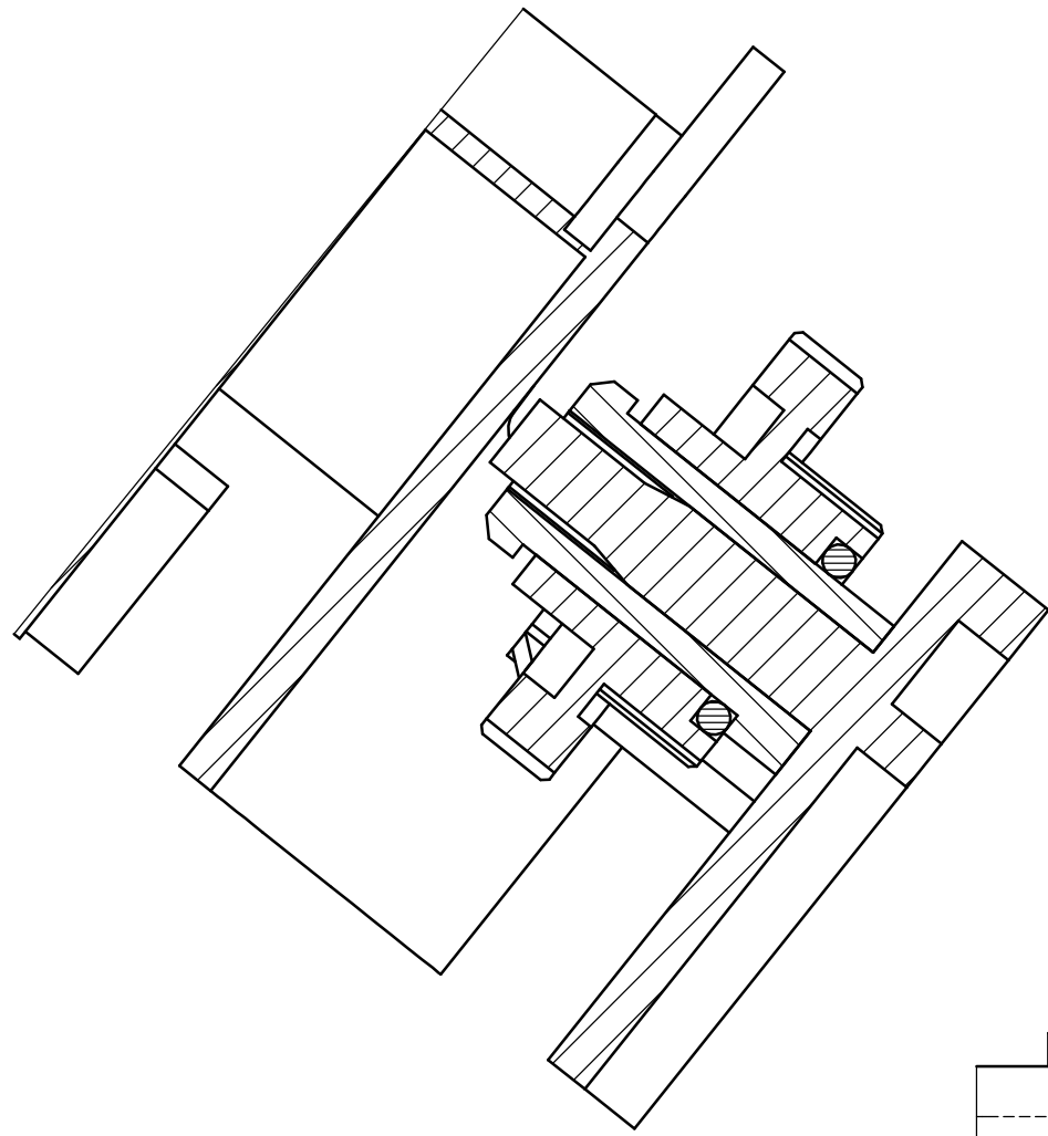
COUPE B-B
