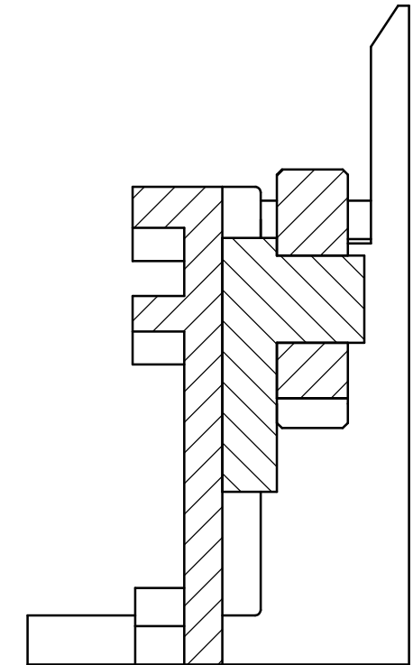
COUPE A-A
